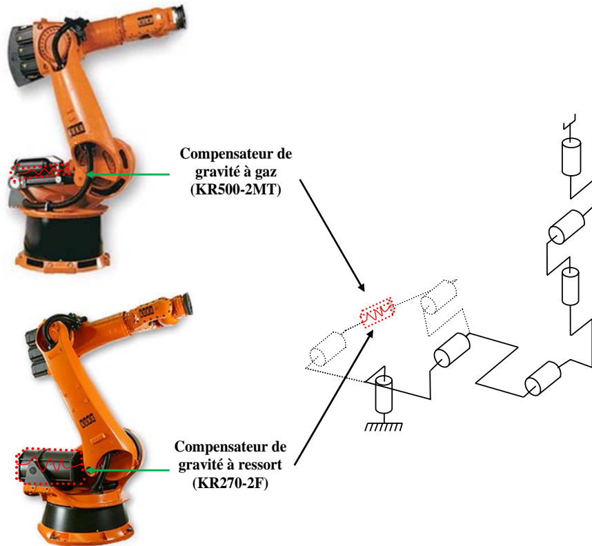
Figure 6: emplacement du compensateur de gravité sur les Kuka KR270-2F et KR500-2MT
