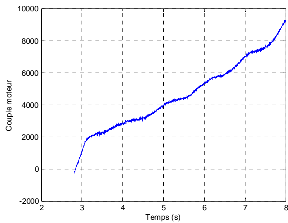
Figure 24: Couple mesuré, axe 2
