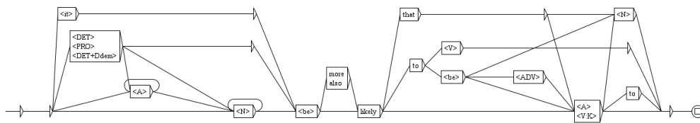
FIG. 8 – Le motif likely.grf.
