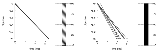
32.4 EBLNS
