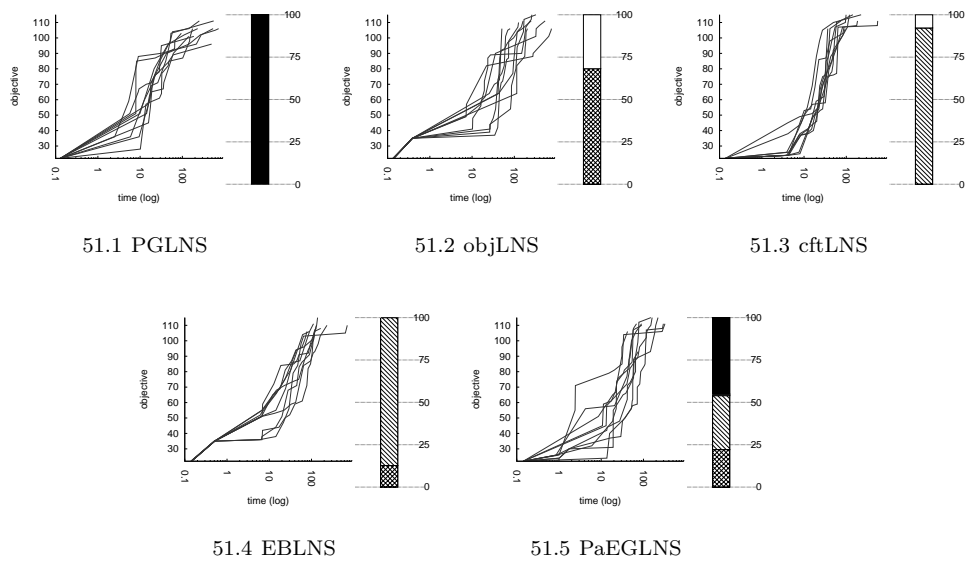
Fig. 51 pc_32-4-8-2.
