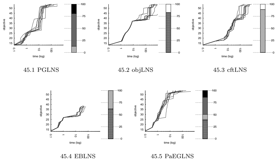
Fig. 45 pattern_set_mining_k2_german-credit.
