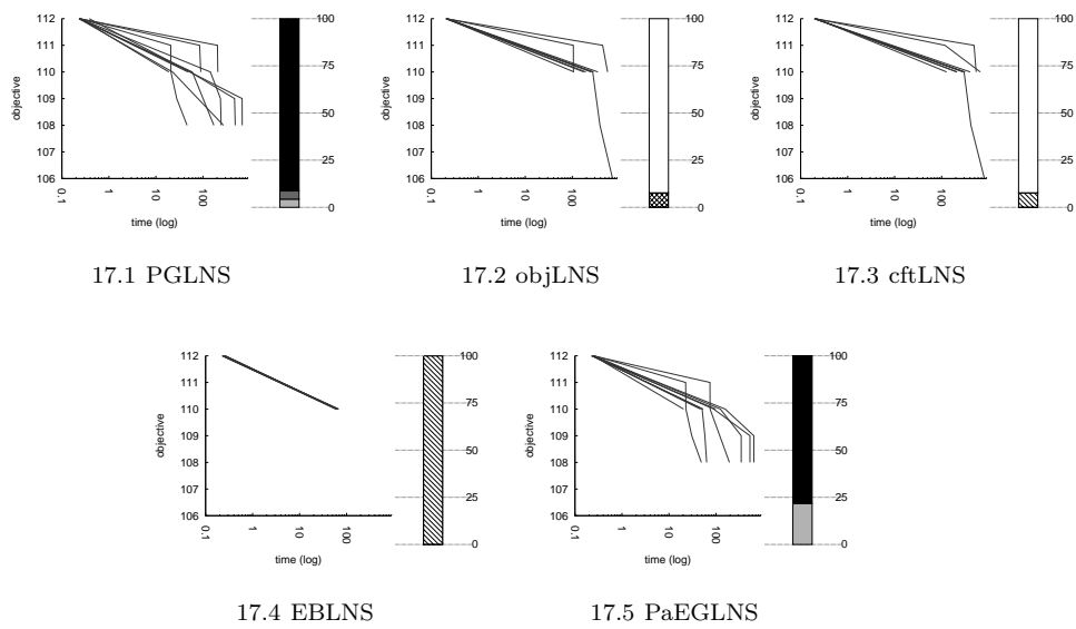
Fig. 17 cars_cars_90.05.
