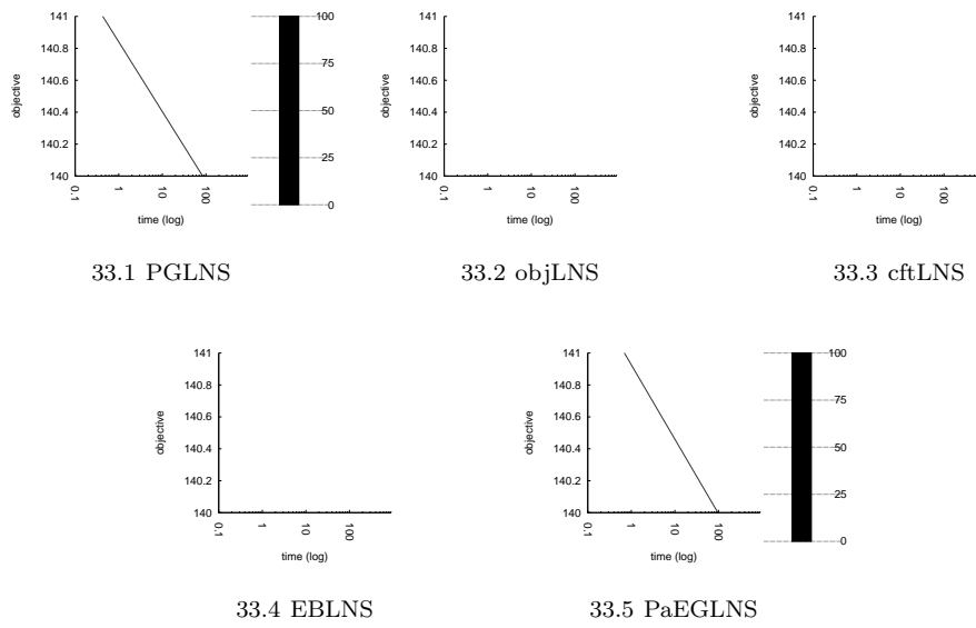
Fig. 33 vrp_A-n38-k5.vrp.
