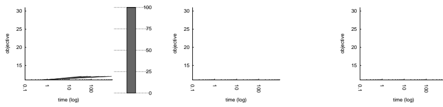
47.1 PGLNS
