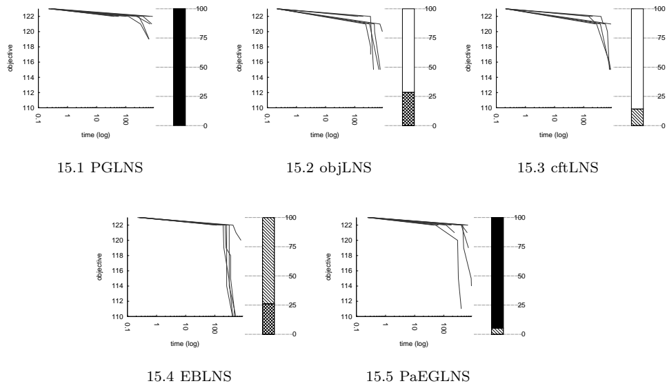
Fig. 15 cars_cars_26.82.
