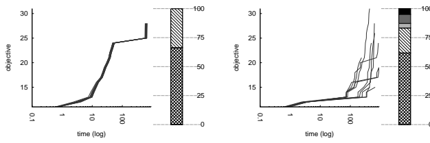
47.4 EBLNS
