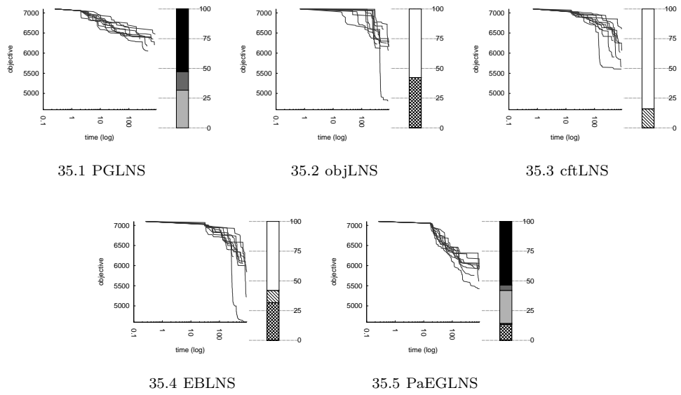
Fig. 35 vrp_B-n51-k7.vrp.
