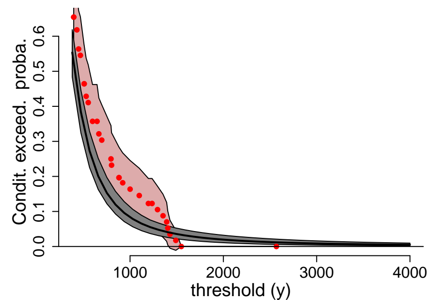
P( Ales > y | Anduze > 520 )
