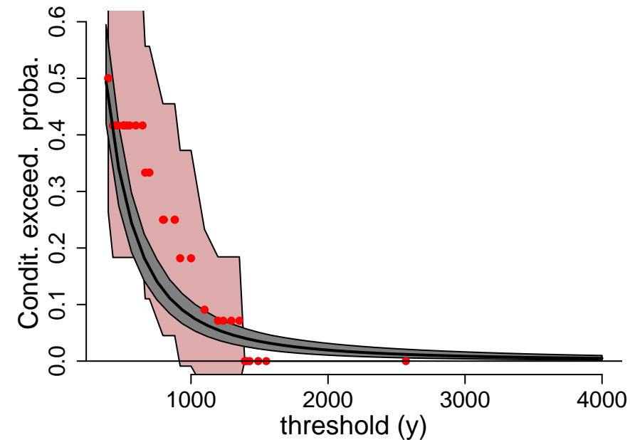
P( Ales > y | St Jean > 300 )
