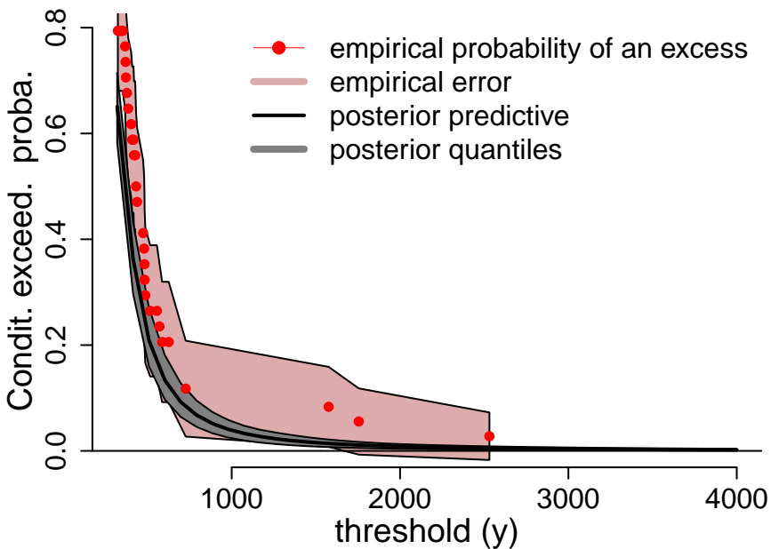
P( Mialet > y | St Jean > 300 )
