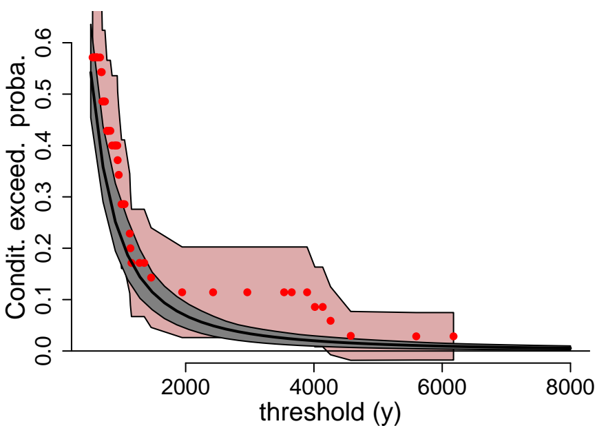
P( Anduze > y | Mialet > 320 )
