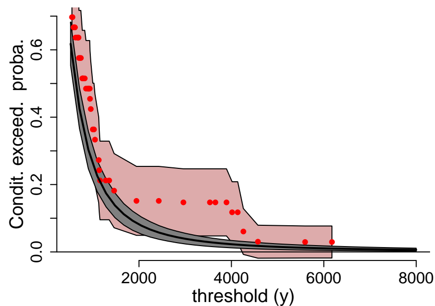
P( Anduze > y | St Jean > 300 )
