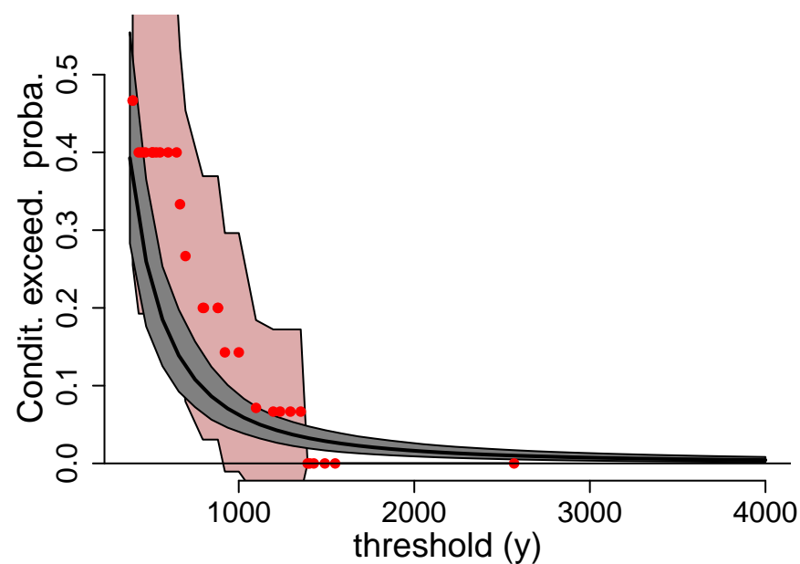
P( Ales > y | Mialet > 320 )
