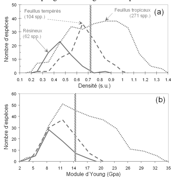
Figure 3. Distribution (en nombre d'espèces) de la densité (a) et du module d'Young (b) par grandes catégories. La ligne verticale représente la moyenne sur toutes les espèces.
