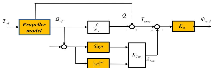
Figure 6 : Exemple d'application de la commande par mode de glissement pour le mode mécanique.
