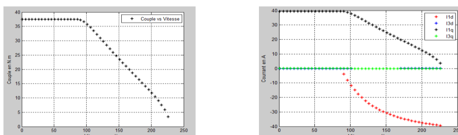
Figure 6: Forme d'onde du couple et des courants pour une machine à FEM sinusoïdale sans injection de courant d'harmonique 3 (courants sinusoïdaux)
