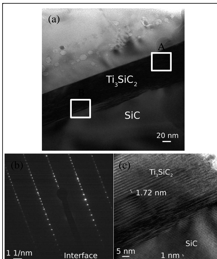
Figure 4 : (a) Image TEM montrant l'interface entre \text{Ti}_3\text{SiC}_2 et 4H-SiC (0001) après recuit à 1000°C/10'. (b) Diffraction électronique de la zone (A) sélectionnée, cette diffraction correspond à la phase \text{Ti}_3\text{SiC}_2 . (c) HRTEM réalisée sur la région (B).
