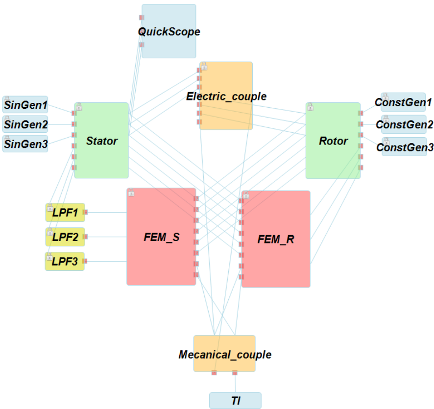
FIGURE 61 : MODÈLE DE LA MACHINE ÉLECTRIQUE.
