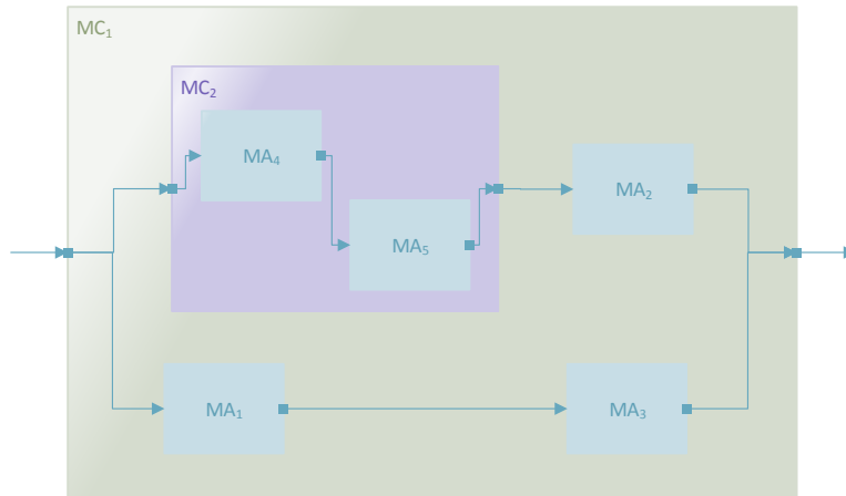
FIGURE 5 : EXEMPLE D'UN MODÈLE COUPLÉ DEVS.
