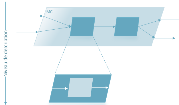
FIGURE 6 : NIVEAU DE DESCRIPTION DANS DEVS.
