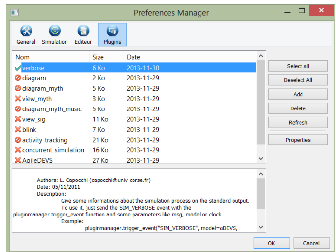
FIGURE 56 : GESTIONNAIRE DE PLUGINS GLOBAUX.
