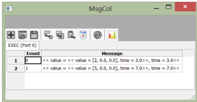
FIGURE 20 : FENÊTRE DE RÉSULTATS DU MODÈLE MSGCOL.
