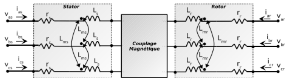
FIGURE 58 : MODÈLE ORIENTÉ CIRCUIT DE LA MACHINE À INDUCTION TRIPHASÉE.
