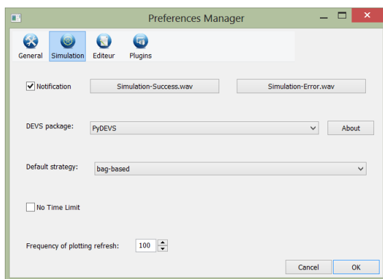
FIGURE 29 : PRÉFÉRENCE DE SIMULATION.
