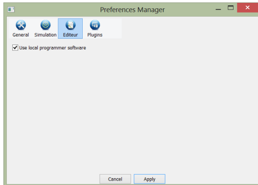
FIGURE 30 : PRÉFÉRENCES D'ÉDITION.
