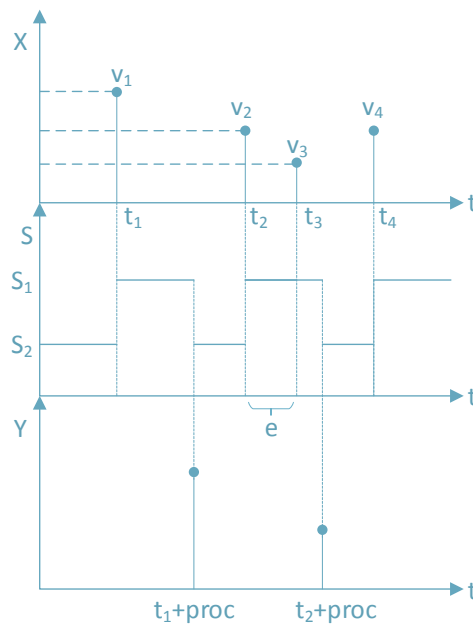
FIGURE 4 : TRAJECTOIRE D'ÉTATS DU MODÈLE EXEC.
