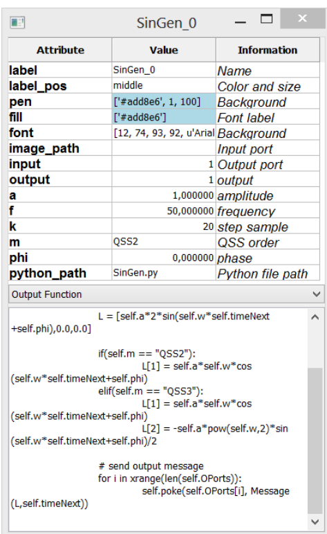
FIGURE 42 : EXEMPLE D'ATTRIBUTS SR LE MODÈLE SINGEN_0.
