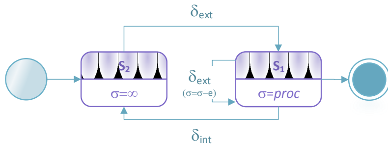
FIGURE 3 : AUTOMATE DU MODÈLE EXEC.
