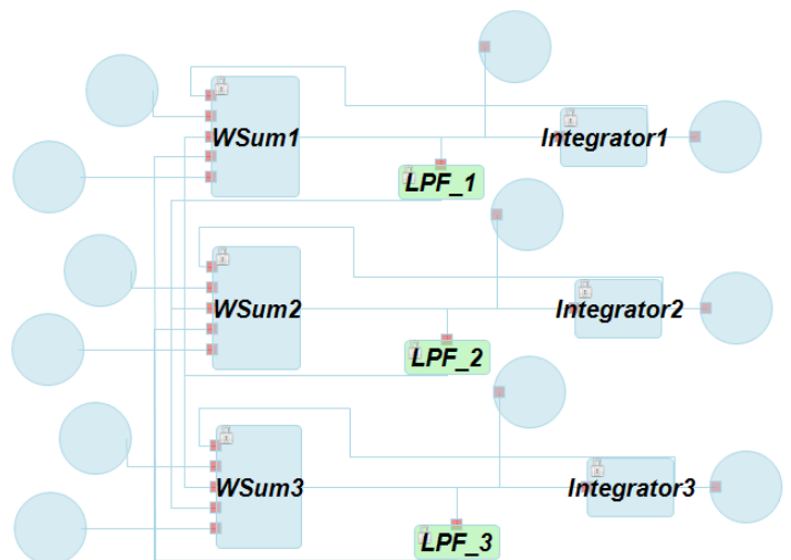
FIGURE 62 : MODÈLE COUPLÉ DU STATOR.
