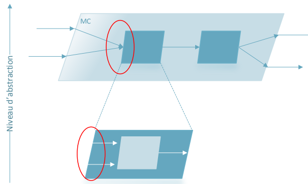
FIGURE 7 : NIVEAU D'ABSTRACTION DANS DEVS.
