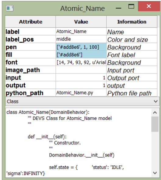
FIGURE 12 : PROPRIÉTÉS D'UN MODÈLE ATOMIQUE.
