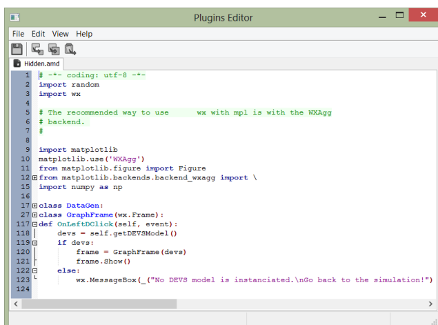
FIGURE 41 : EDITION DU CODE PYTHON D'UN PLUGIN.
