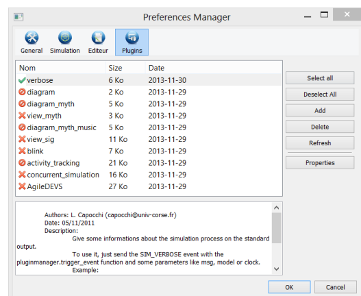
FIGURE 31 : PRÉFÉRENCES DES PLUGINS.
