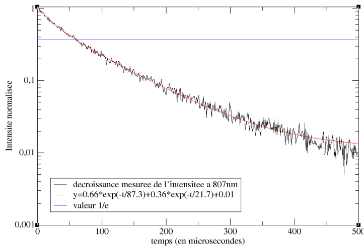
Fig. 2 : Mesure de la décroissance de la fluorescence à 807 \text{ nm} dans la fibre. Le déclin est ajusté avec deux exponentielles. Le trait horizontal correspond à la valeur en 1/e .
