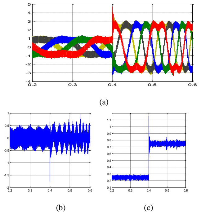
Figure.8. Configuration sans défaut (a) courant dans les phases 1,2, 3 4,5 (b) l'erreur dans la phase 2 (c) couple
