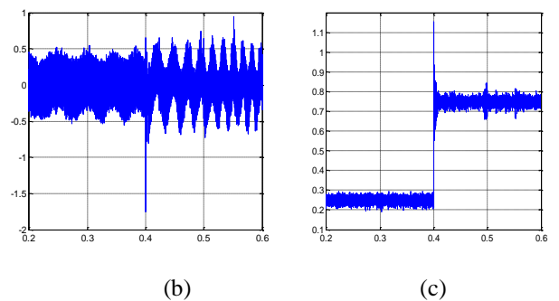
Figure.8. Configuration sans défaut (a) courant dans les phases 1,2, 3 4,5 (b) l'erreur dans la phase 2 (c) couple
