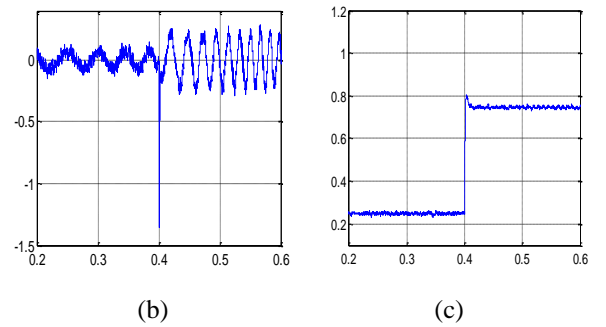
Figure.7. Configuration sans défaut (a) courant dans les phases 1,2, 3 4,5 (b) l'erreur dans la phase 2 (c) couple
