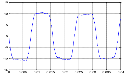
Figure 3 : Relevé expérimental d'une FEM à 1250 tr/mn
