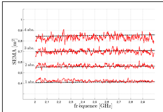
Fig. 2 Evaluation de la SEMA associée à 1,2,ou 3 ou 4 absorbants. Les courbes oscillantes correspondent aux estimations expérimentales selon (11). Les courbes en traits pointillés correspondent à l'évaluation théorique selon (3)
