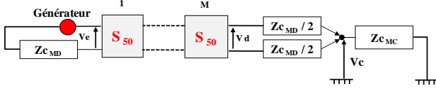
Fig.3 : Simulation d'une ligne torsadée écrantée.
