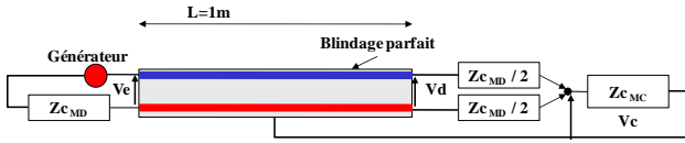
Fig.6 Modèle comportemental de l'ouverture métallique
