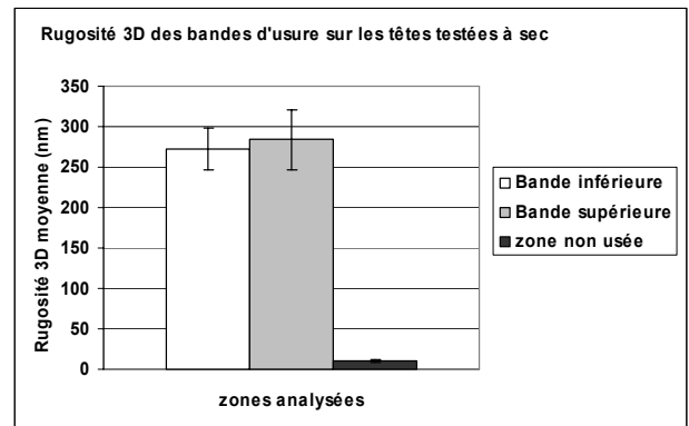
Figure 7. Rugosité des bandes d'usure sur les têtes fémorales, essais à sec.
