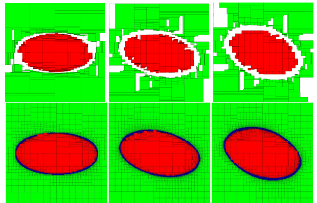
FIGURE 10 – Section 2D d'un pavage 3D obtenu pour le cas 7. De gauche à droite : les angles de rotation sont 0, 0.4 et 0.7. Haut : avec RSOLVER. Bas : avec notre algorithme.
