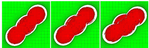
FIGURE 11 – Section 2D d'un pavage 3D obtenu pour le cas 8. De gauche à droite, les angles de rotation sont 0, 0.1 et 0.3. Ce pavage est calculé avec notre algorithme.
