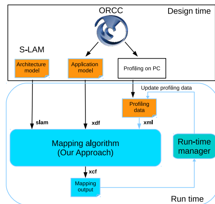
FIGURE 1. Vue d'ensemble de notre flot de déploiement d'acteurs dataflow
