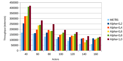
FIGURE 2. Débit pour des réseaux variant de 40 à 160 acteurs sur une plateforme de 8 processeurs
