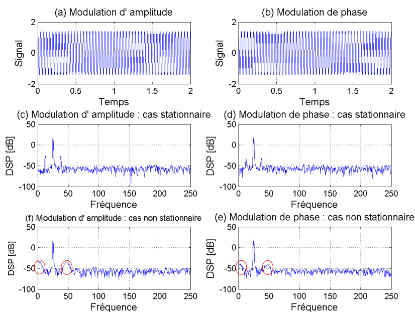
Figure 2. Signaux modulés en phase et en amplitude et leurs périodogramme
