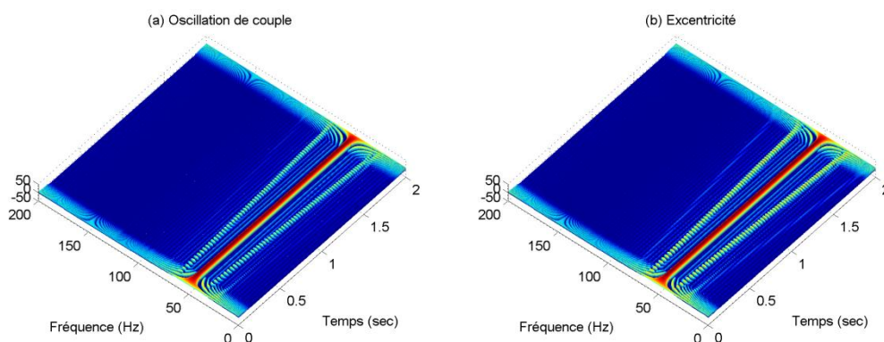
Figure 5. Distribution de Wigner-Ville d'une génératrice en défaut
