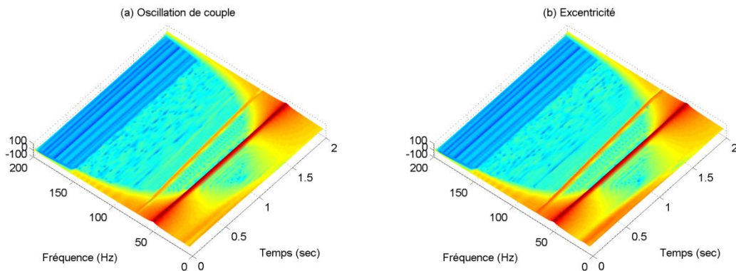
Figure 4. Scalogramme d'une génératrice en défaut
