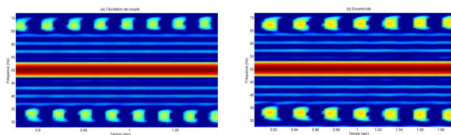
Figure 6. Distribution de Wigner-Ville : (a) Modulation de phase, (b) Modulation d'amplitude
