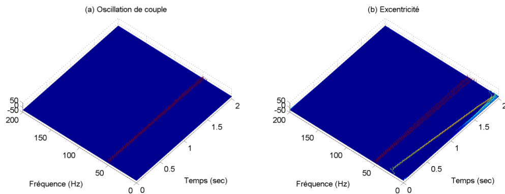
Figure 7. Transformée d'Hilbert-Huang d'une génératrice en défaut
