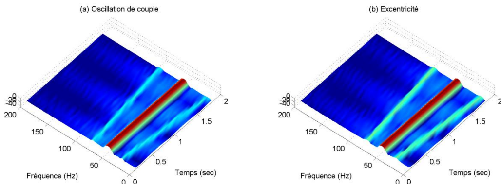
Figure 3. Spectrogramme d'une génératrice en défaut
