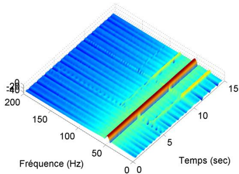
(b) Spectrogramme
