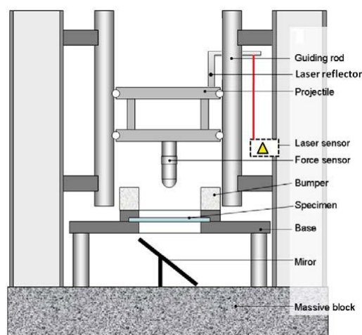
Figure 1 : schéma du dispositif expérimental ; la tour de chute.
