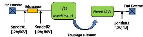
Fig. 5: Couplage entre structures basiques (NWell)
