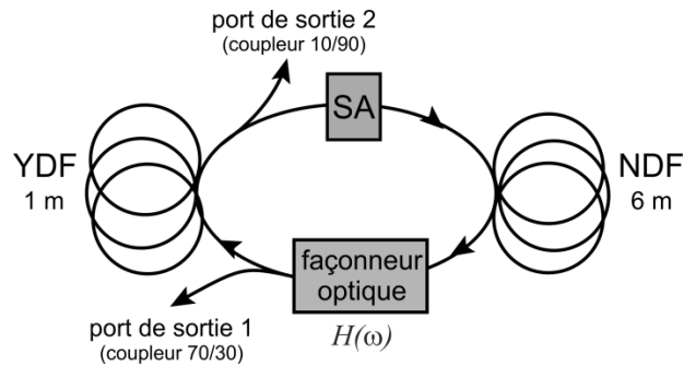
Fig. 1 : Vue schématique de la cavité laser fibrée considérée.
