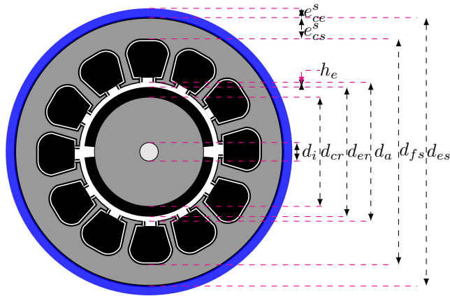
Fig 2 – Coupe transversale du moteur synchrone utilisé
