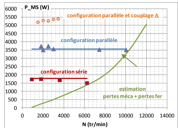
Fig.16: Puissance maximale convertible pour les trois configurations et indication de la somme des pertes mécaniques et des pertes fer.
