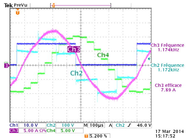
Fig.13: Point de fonctionnement à puissance maximale, en configuration parallèle à 3600 tr/min.
