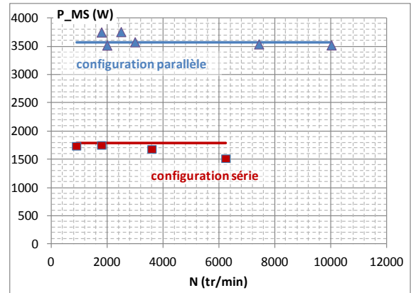
Fig.12: Evolution de la puissance maximale convertie en fonction de la vitesse de rotation pour les deux configurations.
