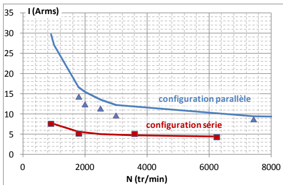
Fig.11: Evolution de la valeur efficace des courants absorbés par la machine électrique en fonction de la vitesse de rotation pour les deux configurations.
