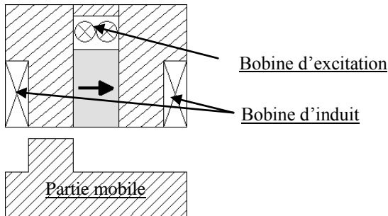
Fig.2: Présentation d'une cellule élémentaire.
