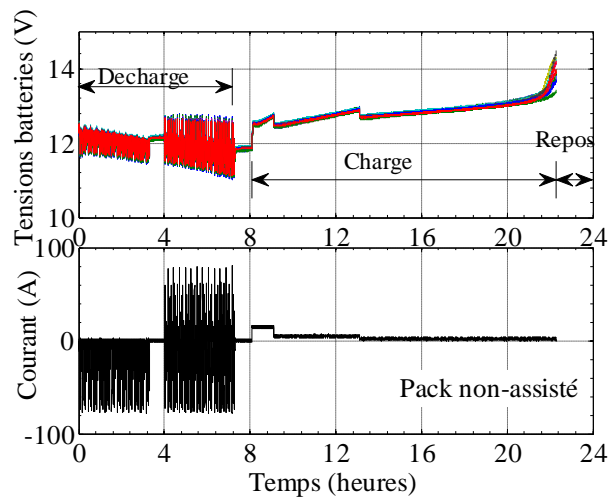
Fig.8 Profil de courant journalier appliqué (mesures)
