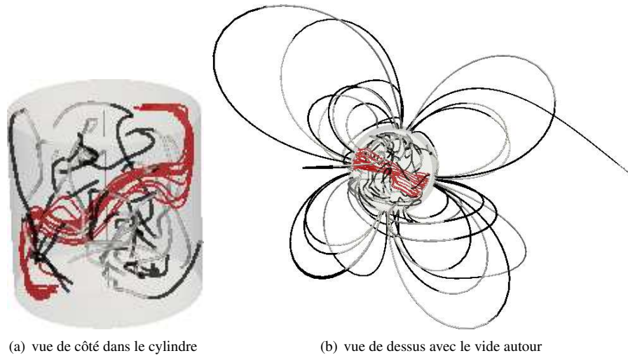
Fig. 2. Vue instantanée à t = 241 pour Re = 1200 , Rm = 2400 montrant des lignes de vorticités (rouge) et des lignes de champ magnétique colorées par la composante axiale H_z .
