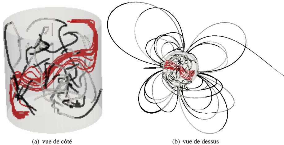
FIGURE 2 – Vue instantanée à t = 241 pour Re = 1200 , Rm = 2400 montrant des lignes de vorticité (rouge) et des lignes de champ magnétique colorées par la composante axiale H_z .
