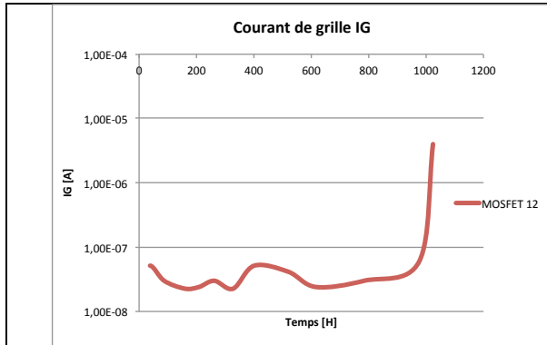
Figure 8 : Courant de grille en fonction du temps
