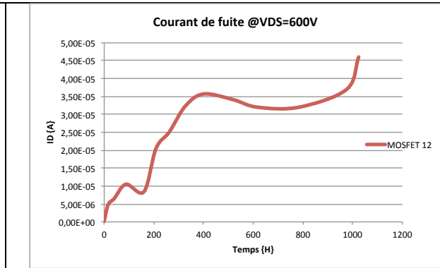
Figure 9 : Courant de fuite en fonction du temps
