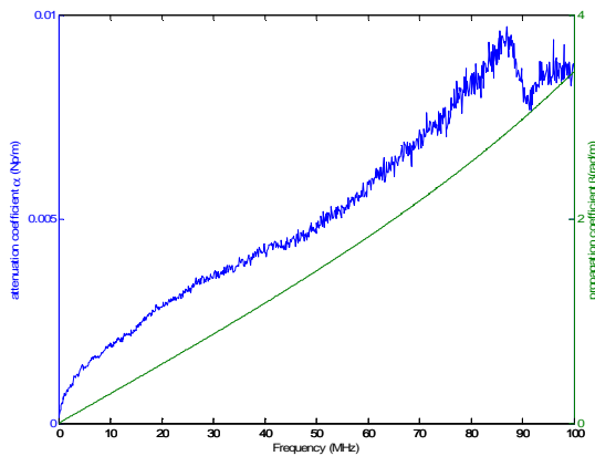
Fig. 15 Coefficient de propagation \gamma = \alpha + j\beta des cables utilisés
