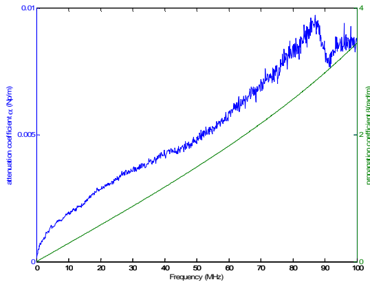
Fig.15 Coefficient de propagation \gamma=\alpha+j\beta des câbles utilisés
