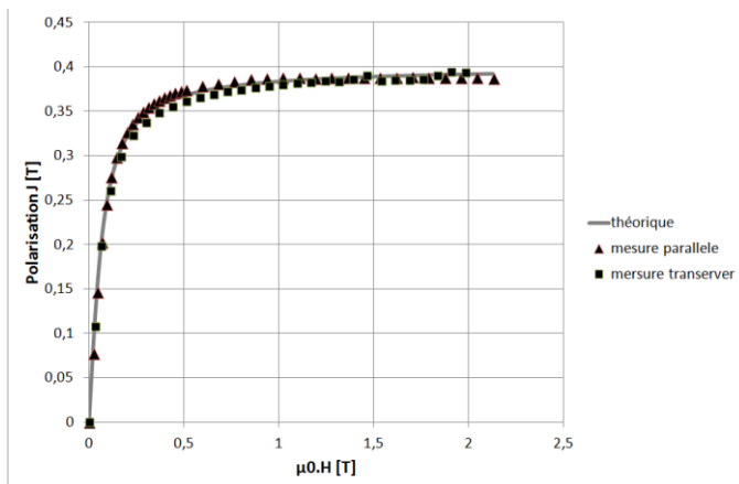
Fig.16. Comparaison des courbes J(H) théorique et mesurées par les deux méthodes.
