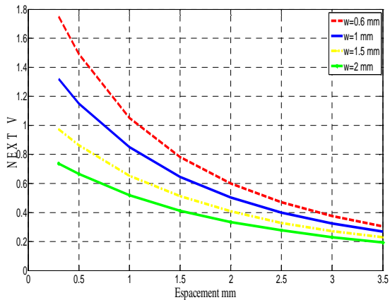
Fig 12. NEXT pour différentes largeurs de piste
