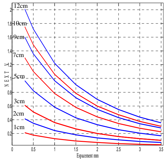
Fig 14. NEXT pour différentes longueurs de piste
