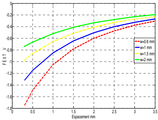
Fig 13. FEXT pour différentes largeurs de piste
