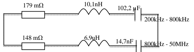
Fig 5. Modèle Spice de XCap
