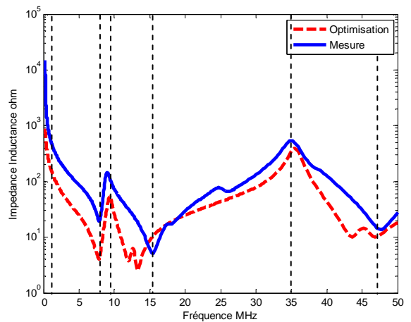
Fig 6. Impédance de XInd
