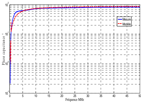
Fig 9. Phase de l'impédance XCap
