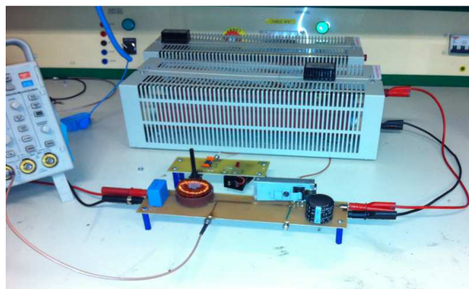
Fig 1. Photographie d'un hacheur survolteur
