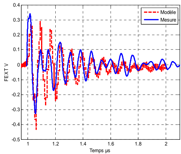
Fig 11. FEXT par modèle et mesure
