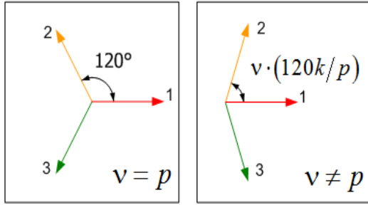
Figure 2: Position relative des axes magnétiques des trois phases en fonction du rang harmonique
