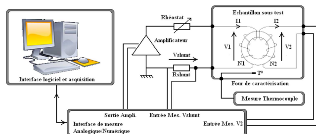
Fig. 1. Schéma de principe de la mesure du cycle B(H) à l'hystérésigraphe.
