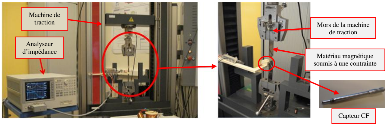
Figure 3 : Banc de mesure
