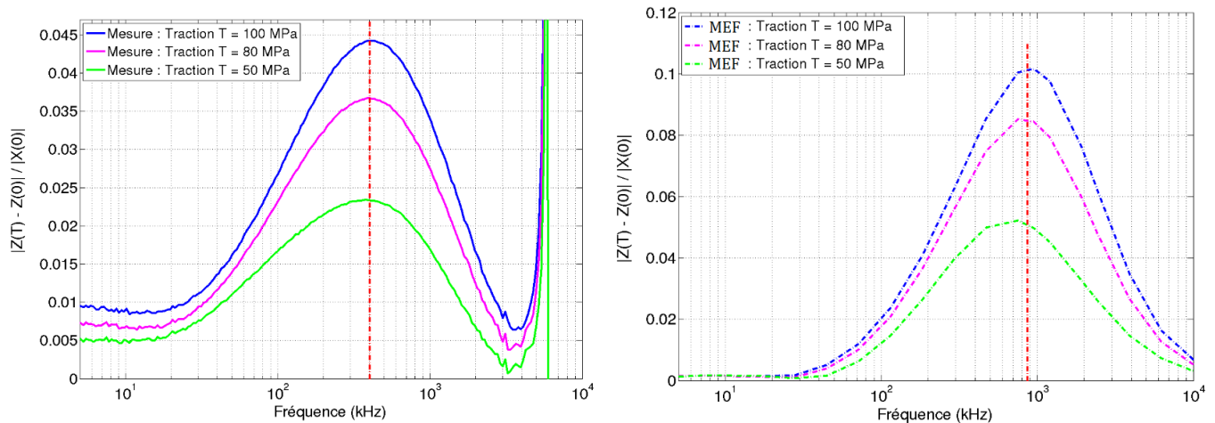
Figure 5 : Variation relative d'impédance pour différentes contraintes de traction T appliquées (50, 80 et 100MPa) en fonction de la fréquence d'excitation du capteur CF : résultats de mesure et calculs numériques
