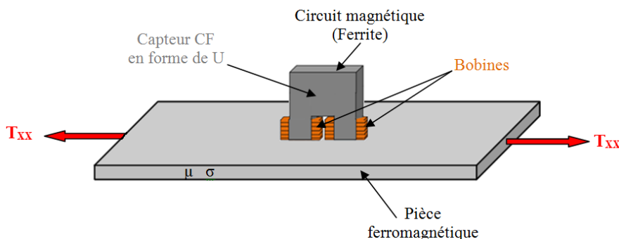
Figure 2 : Configuration CF d'étude
