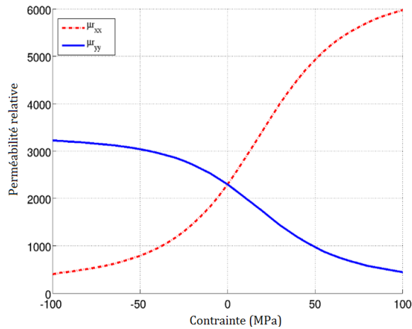
Figure 1 : Composantes du tenseur de perméabilité relative en fonction de la contrainte appliquée pour un alliage de FeCoV (contrainte de traction/compression selon l'axe-X)
