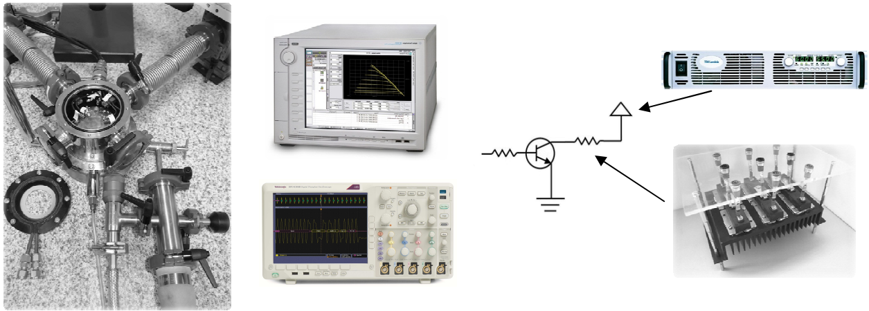
Figure 1: Dispositifs de mesure. De gauche à droite. Cryostat. Traceur Agilent B1505 (haut). Oscilloscope Tektronix DPO4014B (bas). Schéma de mesure en commutation sur charge résistive. Alimentation TDK-Lambda 600V-5.5A (haut). Charge résistive modulable (bas).
