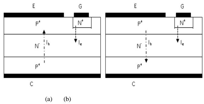
Fig.3 Orientation des courants de trous et d'électrons dans la structure en fonction de la polarité de V_{ce} : V_{ce} > 0 (a) et V_{ce} < 0 (b)
