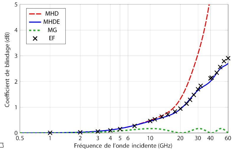
FIGURE 3 – Comparaison des résultats provenant de 3 modèles d'homogénéisation avec ceux provenant d'une modélisation par Eléments Finis.
