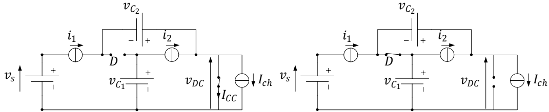
(a) Séquence 1 : séquence de court-circuit de l'onduleur. (b) Séquence 2 : séquence hors état de court-circuit de l'onduleur.
