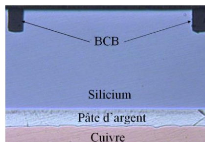
Figure 6 : Vue en coupe de la puce reportée sur substrat après le frittage d'argent.
