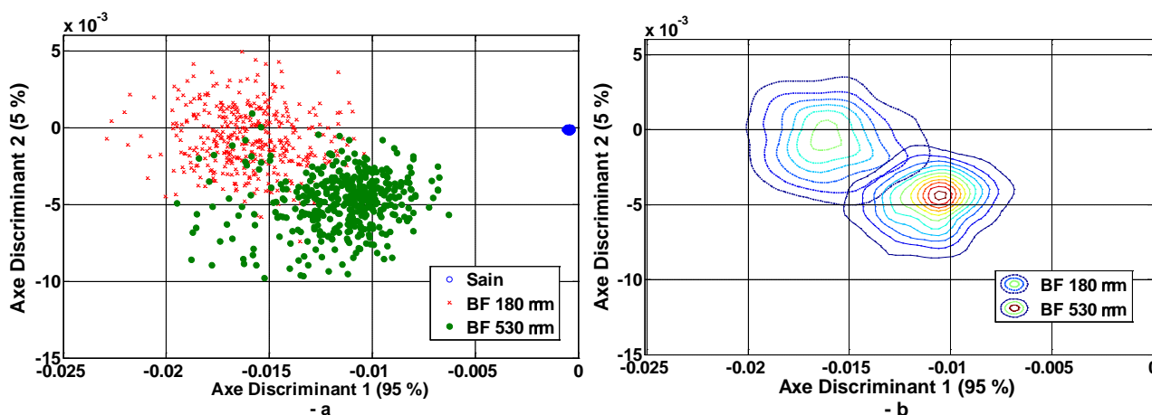
Figure 3 : Discrimination des défauts de billes dans l'espace de l'ADL – a : classes correspondantes – b : contours des niveaux de densité de probabilité estimée pour chaque classe
