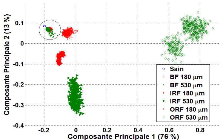
Figure 1 : Classification des défauts de roulements dans le sous-espace principal
