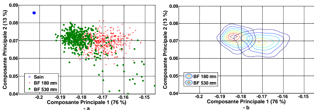
Figure 2 : Discrimination des défauts de billes dans le sous-espace principal – a : classes correspondantes – b : contours des niveaux de densité de probabilité estimée pour chaque classe
