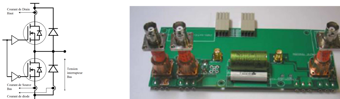
Figure 2 : Implantation des mesures en mode commun du courant et de la tension au niveau du bus continu
