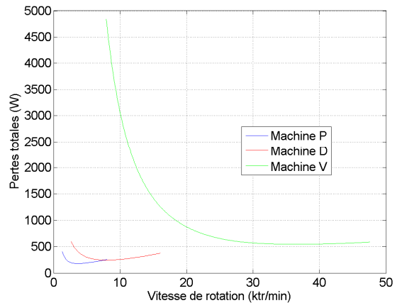
Figure 5. Pertes en fonction de la vitesse de rotation pour trois machines du front
