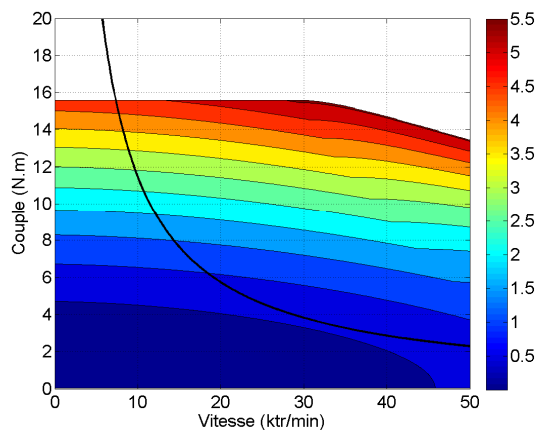
Figure 6. Caractéristique iso-pertes dans le plan couple-vitesse pour la machine V
