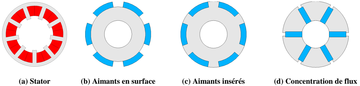
Figure 1 : Architectures de machines étudiées
