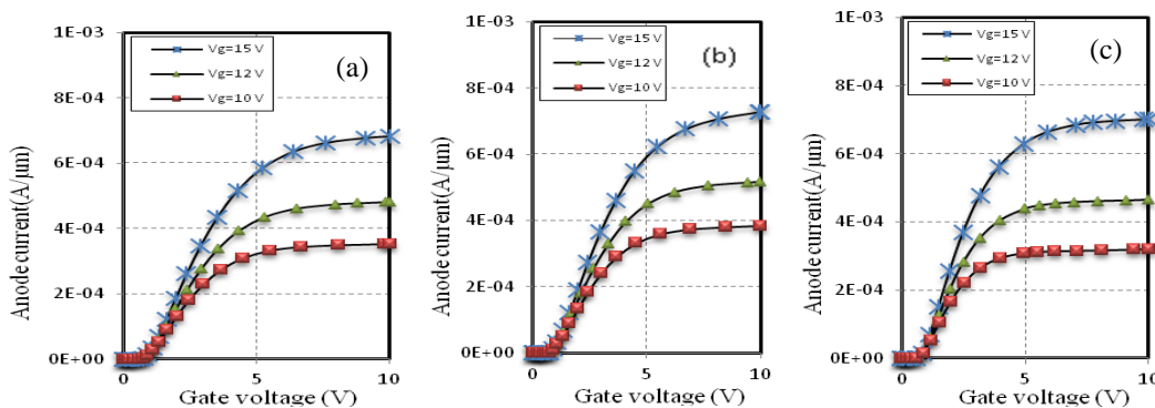
Figure 4 : Caractéristiques de sortie I_A = f(V_{AK}) de (a) l'IGBT standard, (b) l'IGBT-1 et (c) l'IGBT-2
