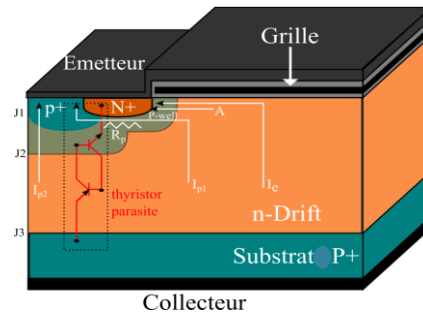
Figure 1 : Latch-up du thyristor parasite dans un IGBT
