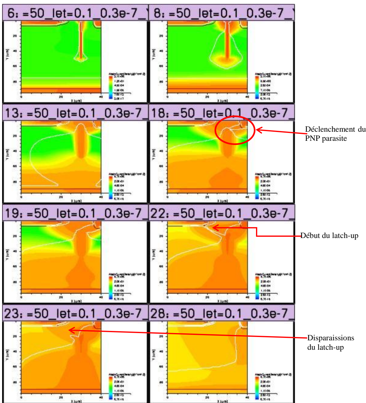
Figure 6 : Distribution du courant à différents instants après l'impact dans l'IGBT-1
