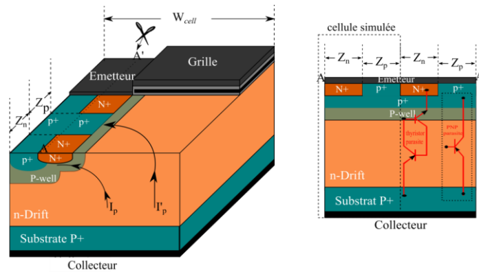
Figure 3 : Représentation schématique de la deuxième modification de la structure par la diffusion de P + dans la région N + émetteur « IGBT-2 » (gauche), coupe 2D suivant AA' (droite)
