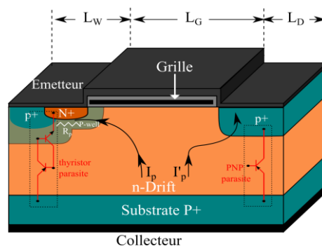
Figure 2 : Représentation schématique de la première modification de la structure par l'ajout d'une diffusion P^+ dans la région intercellulaire (IGBT-1).
