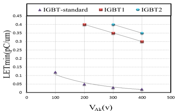
Figure 5 : LET minimal déclenchant un SEB pour différentes polarisations d'un ion lourd provenant de la face avant dans l'IGBT standard, l'IGBT-1 et l'IGBT-2
