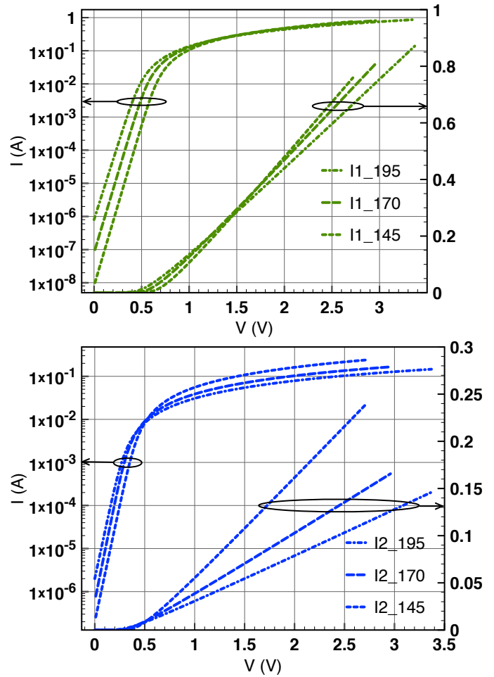
Fig. 8. Branches 1 (en vert) et 2 (en bleu) dissociées du modèle double branche d'un composant d'étude Schottky Ni/SiC à 195°C, 170°C et 145°C.
