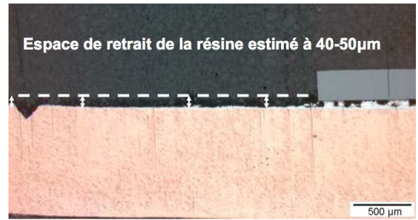
Fig. 7. Illustration de la délaminatation résine/semelle sur une coupe transversale.
