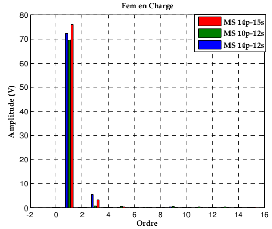
Fig 5 : Force électromotrice MS à double bobinage concentré
