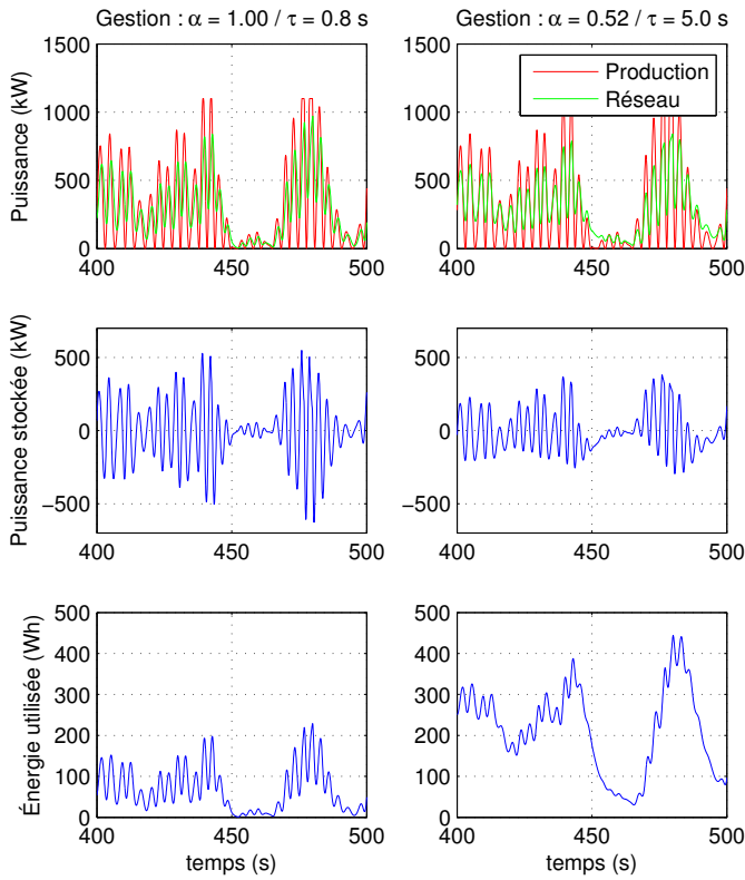
Fig. 7. Lissage d'une production houlogénérée suivant deux couples de paramètres (\alpha, \tau) différents de la loi de gestion : état de mer H_s = 2.5 m, T_p = 8 s (190 kW moyen), P_{lt} = 0.056 dans les deux cas (contrainte de flicker respectée)
