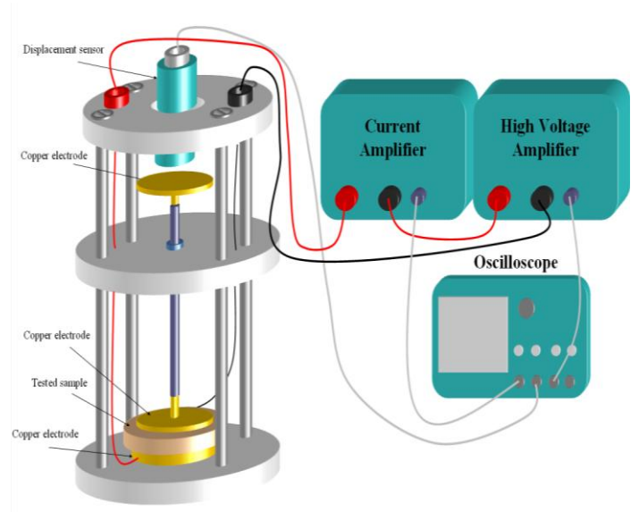
Fig.1Banc de mesure expérimental
