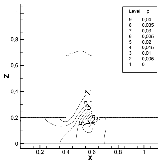
FIGURE 5. Champ de pression de sur une coupe à y=0,1m de la conduite optimisée dans le plan de symétrie XOZ (zoom)
