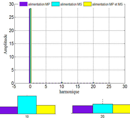
Figure 12 : Contenu harmonique du couple électromagnétique de la machine 20/8/5 (estimation numérique)
